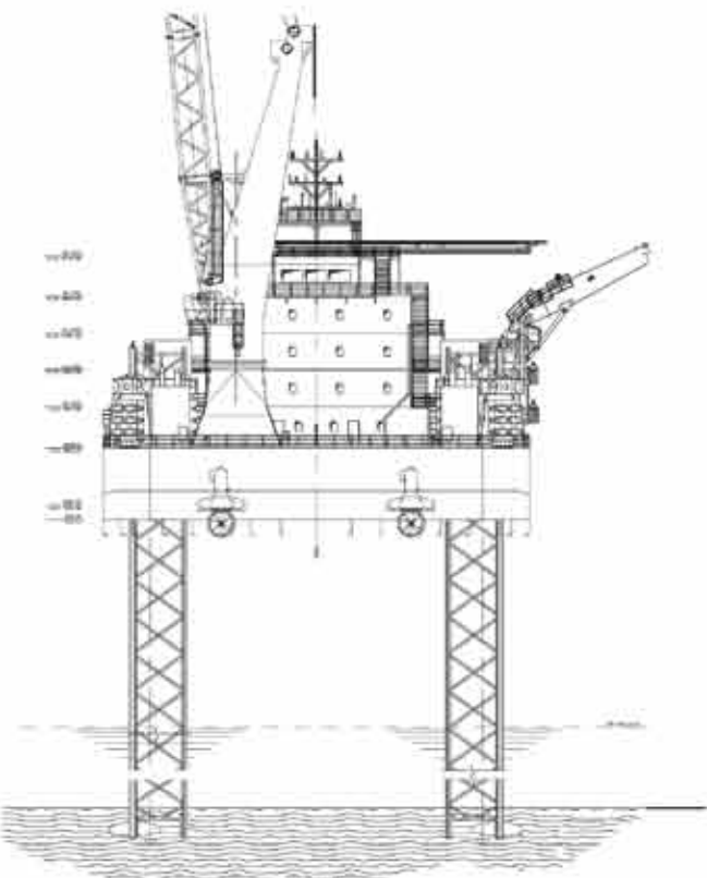
AFTVIEW
